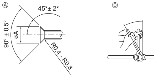
Ⓐ Afsnijmten tromp Ⓑ Aanhaalmoment flensmoer
