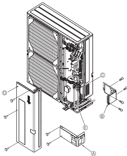
Ⓐ Vordere Leitungsabdeckung Ⓑ Leitungsabdeckung Ⓒ Absperrventil Ⓓ Wartungspult Ⓔ Radius der Biegung : 100 mm - 150 mm
